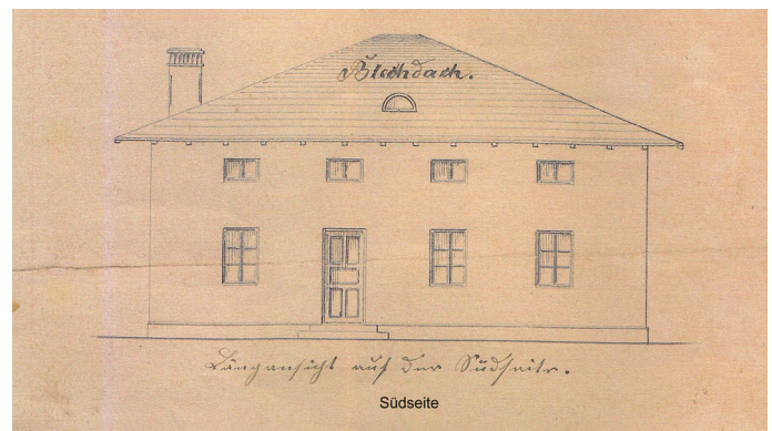
Südansicht des Bräuhaus-Bauplans
